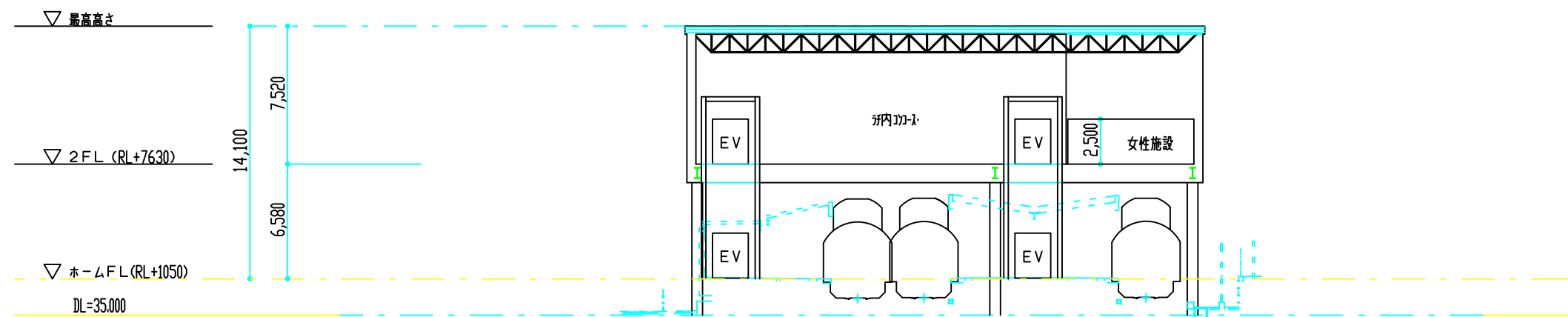
b-b 断面図
