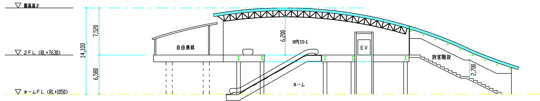
a-a 断面図
