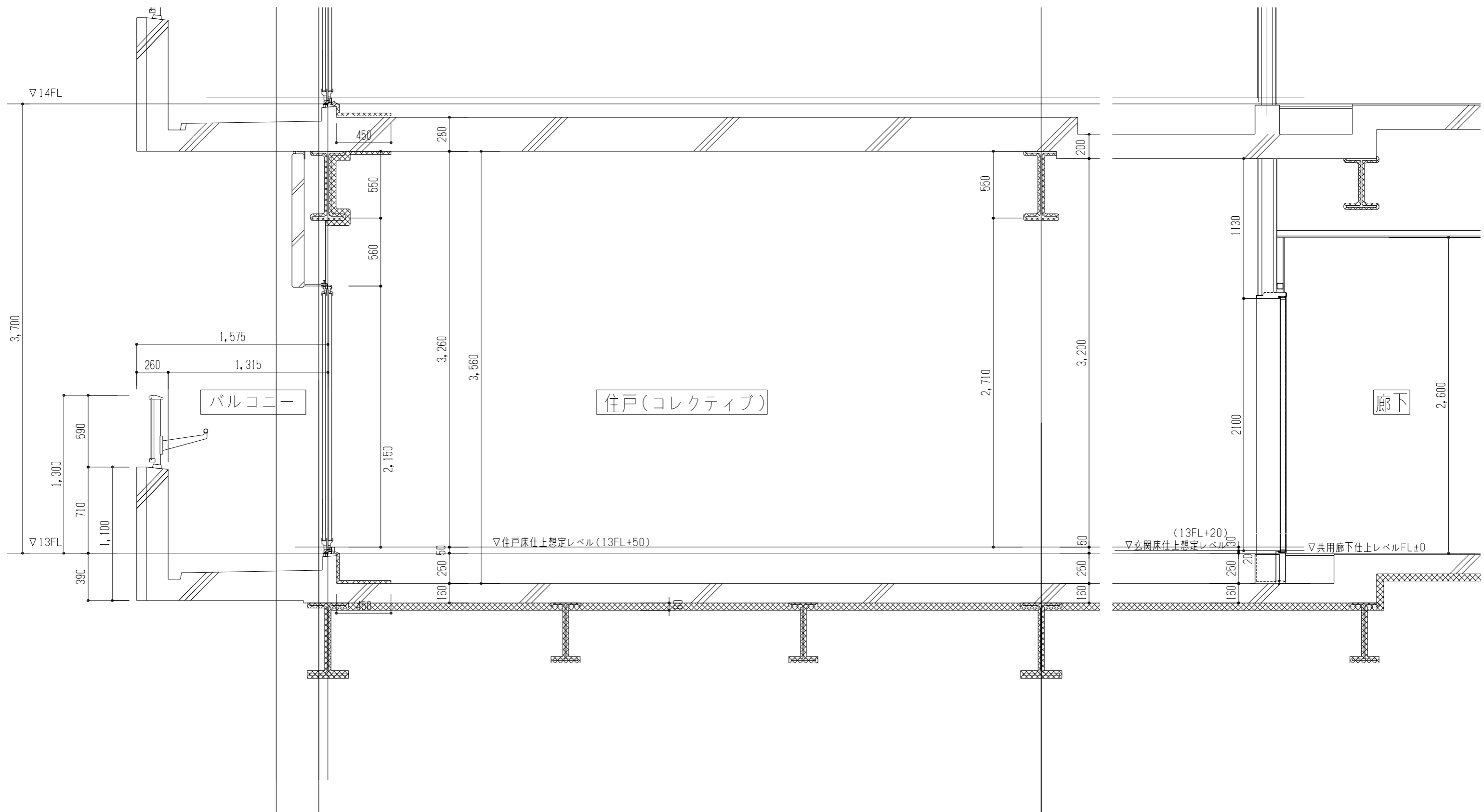
1 13階断面詳細図 (コレクティブ) S=1/30
