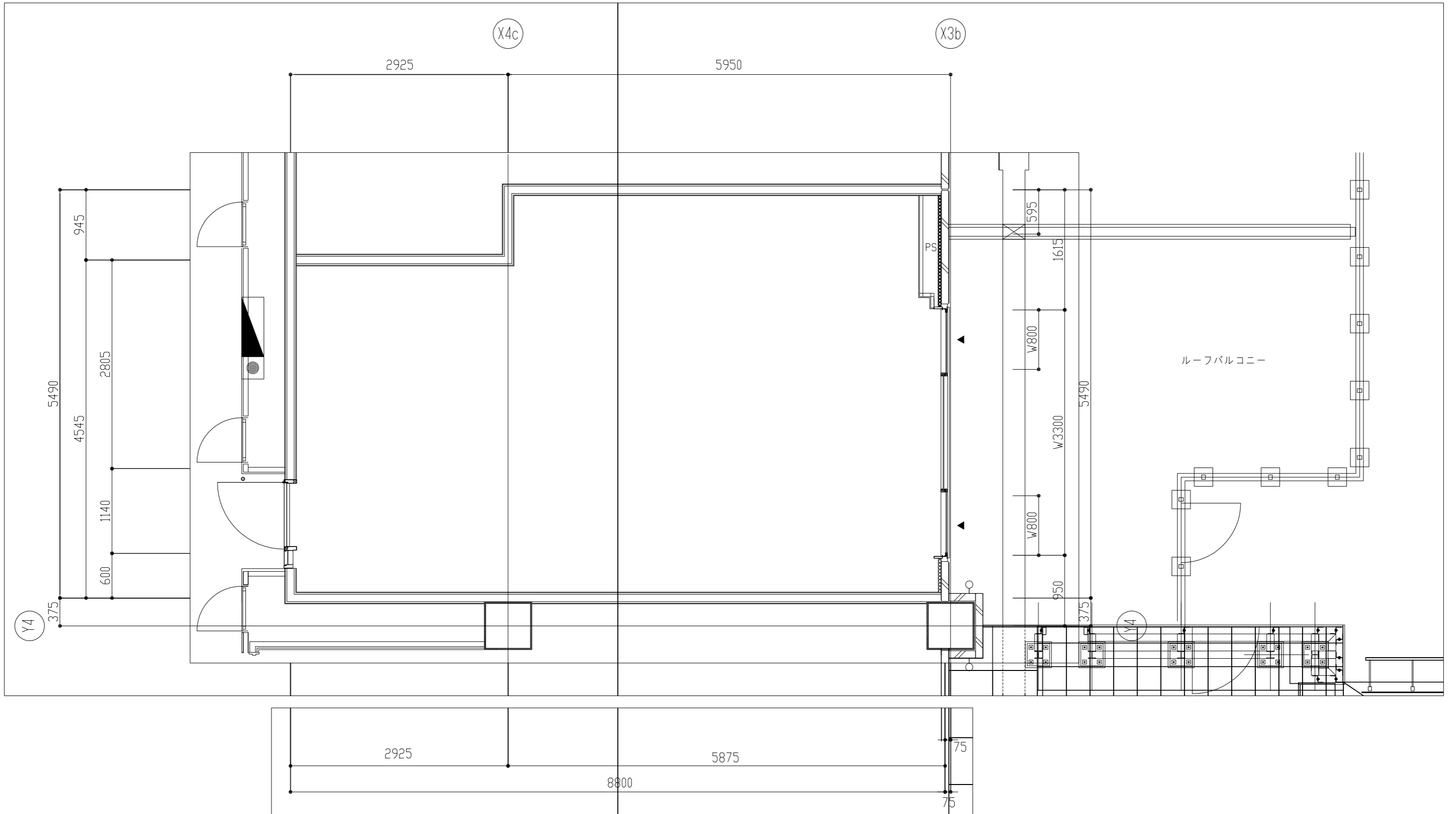
1 平面図 c40Cc S=1/50
