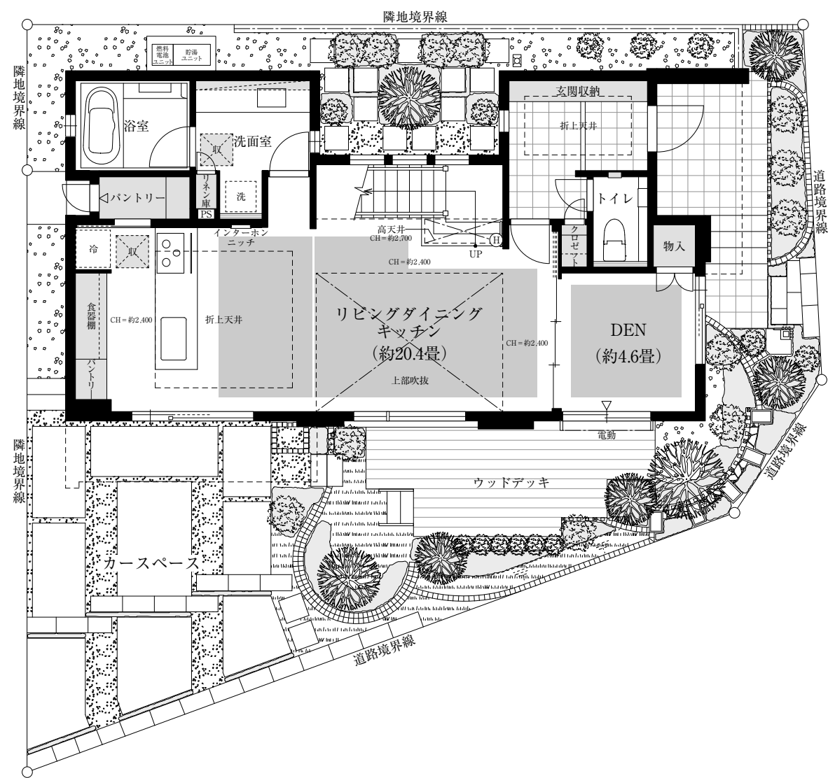
■1階平面図
